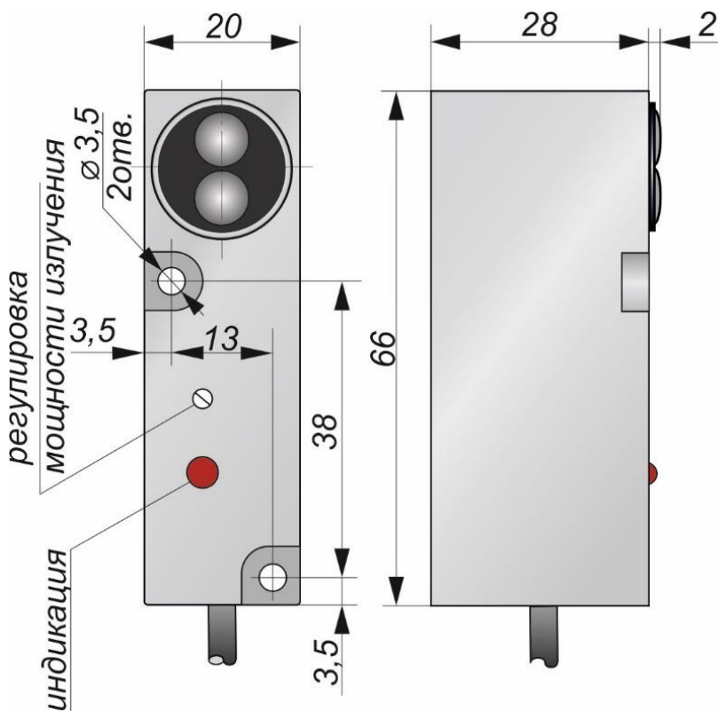
Габаритный чертеж
