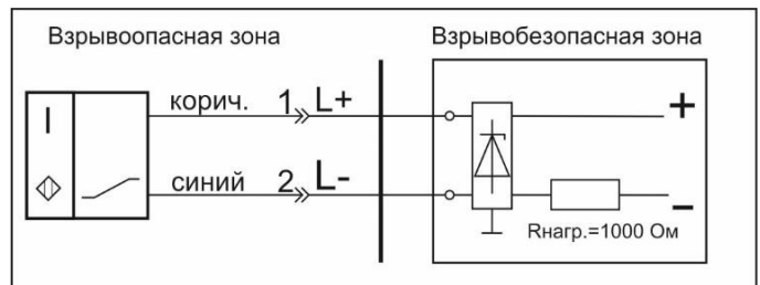
Схема соединения
