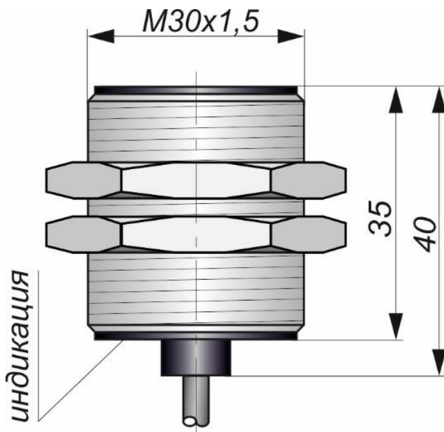
Габаритный чертеж
