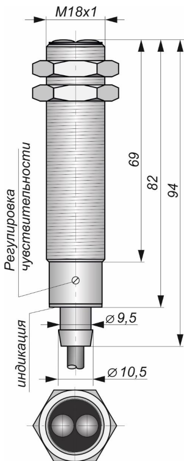
Габаритный чертеж
