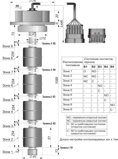
Габаритный чертёж
