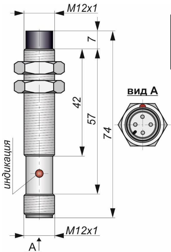
Габаритный чертеж
